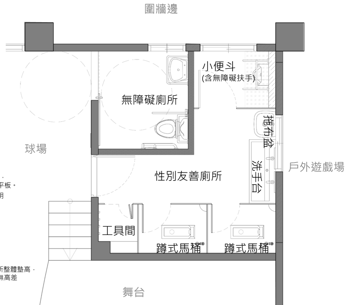
廁所設計平面圖
