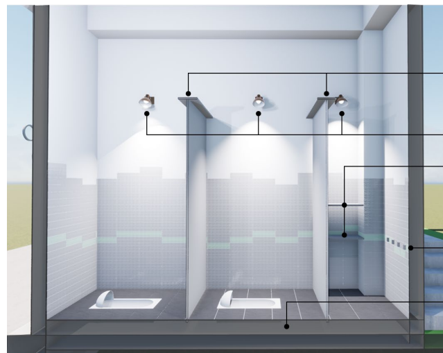
廁間設計： 防偷窺設計、獨立充足照明、增設工具 收納空間、地坪墊高。
