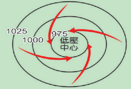
北半球氣旋
